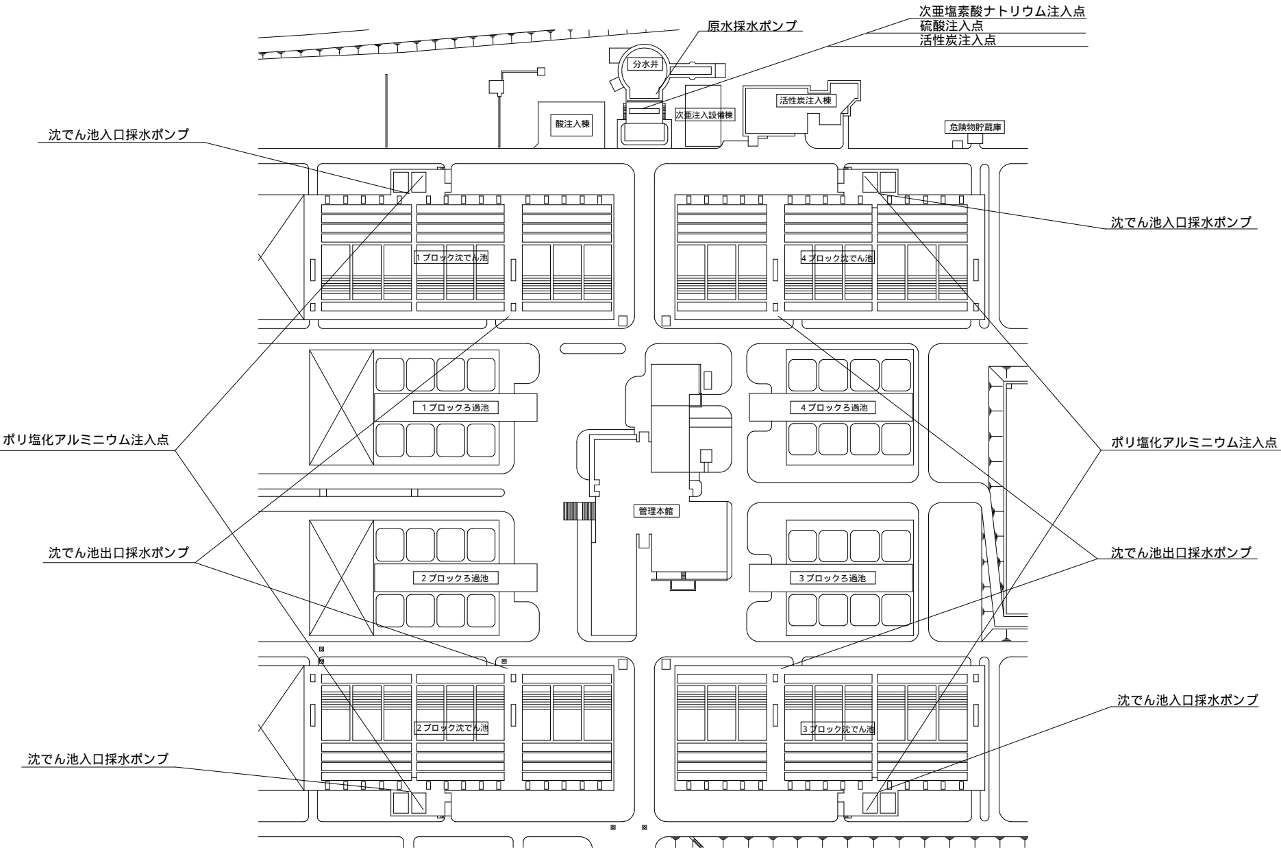
相模原浄水場 全体平面図
