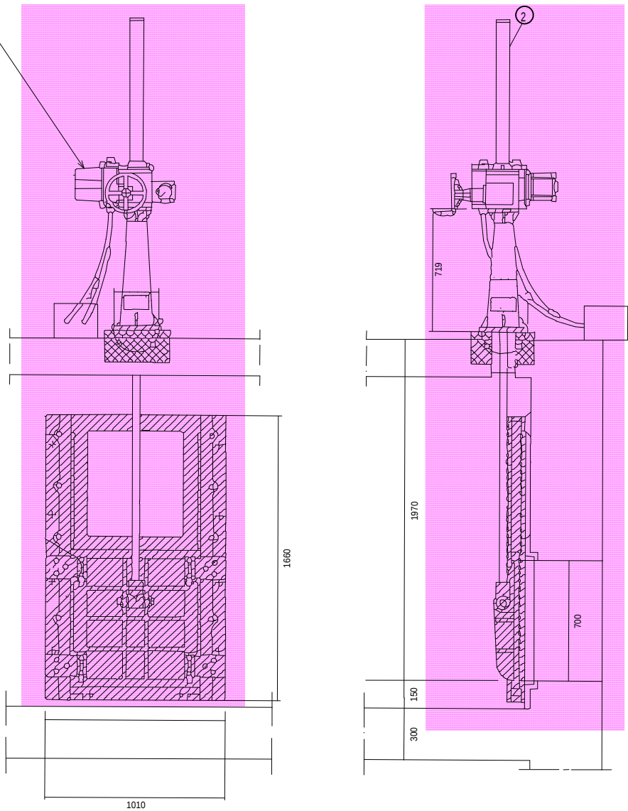
沈でん池 制水扉 断面図
