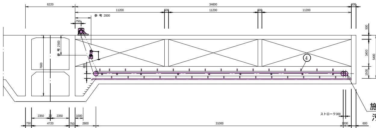
A—A 断面图
