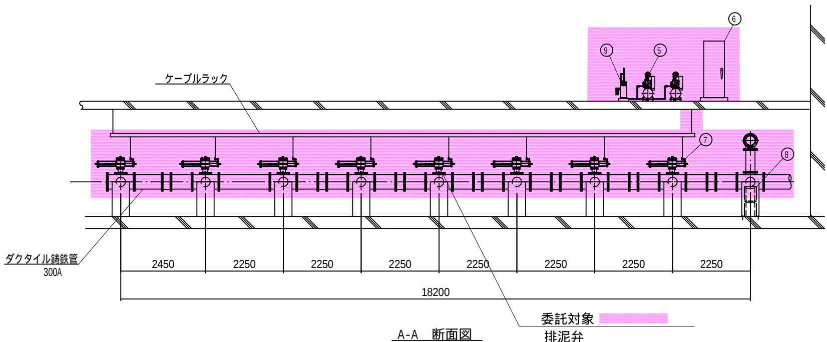
沈でん池 排泥管廊 断面図
