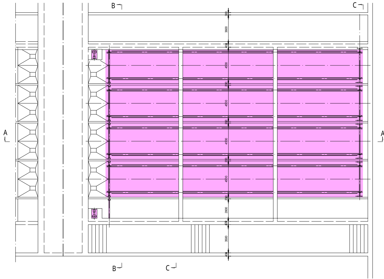
沈でん池 汚泥掻寄機 平断面図
