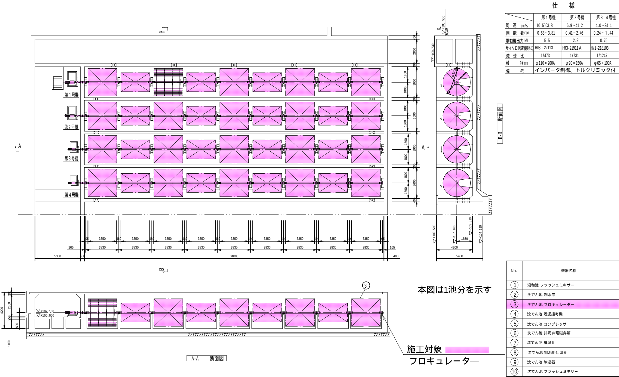
沈でん池 フロキュレーター 平断面図
