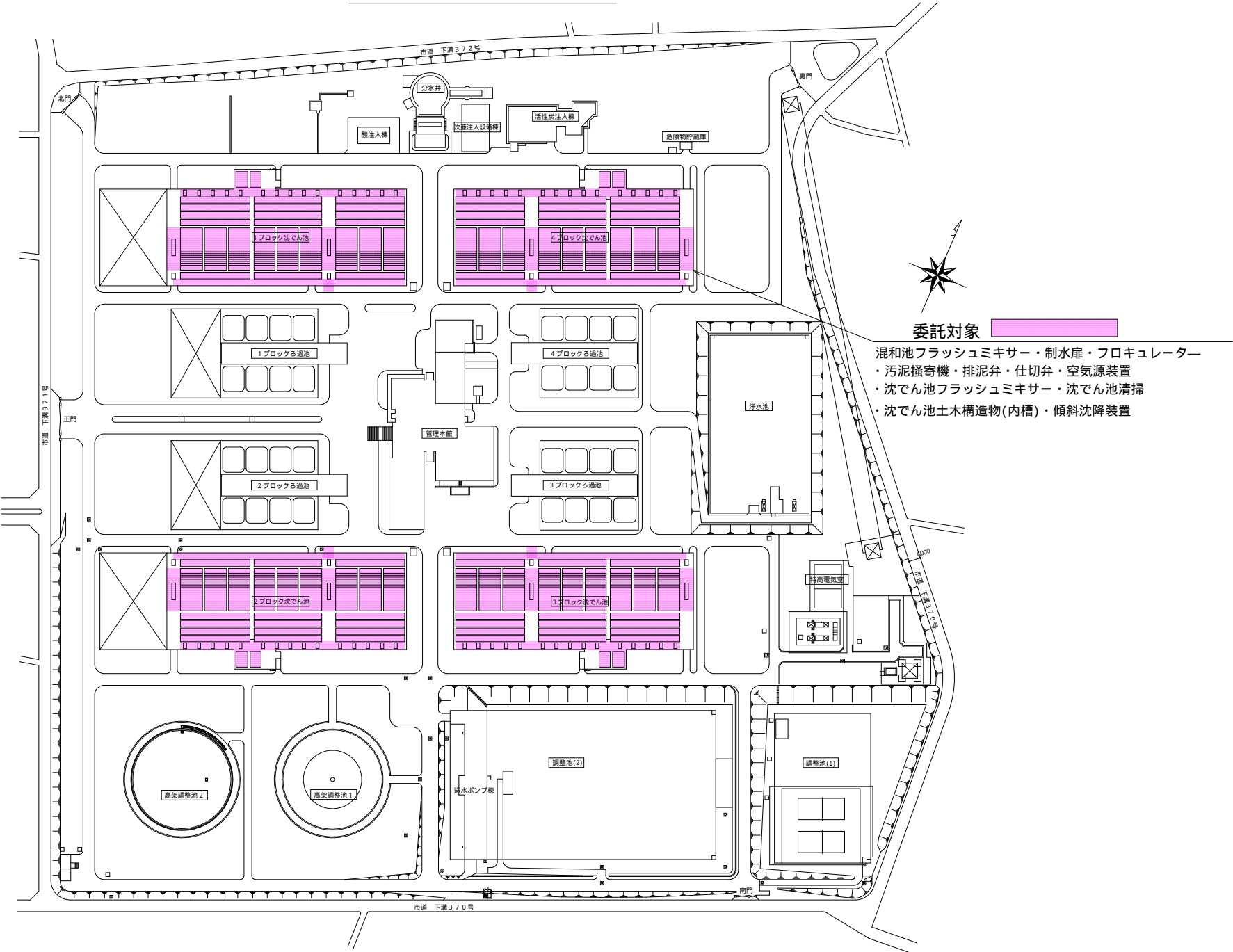
相模原浄水場 全体平面図
