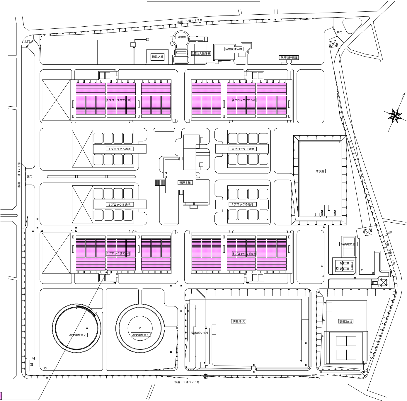
相模原浄水場 全体平面図
