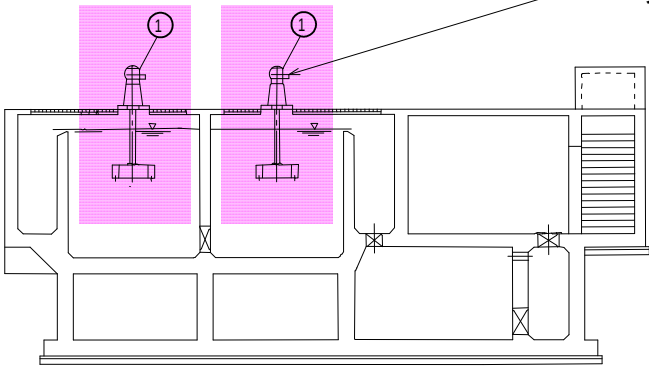
A-A断面図
