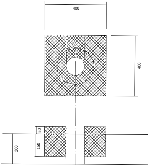
基礎図
