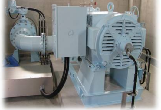
矢指小水力発電設備
